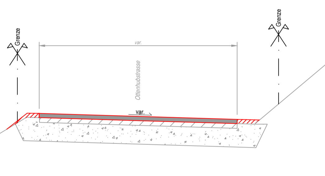
Normalprofil 1 (Hocheinbau)
