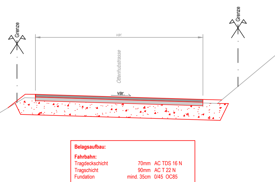
Normalprofil 2 (Fundamentersatz)
